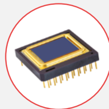
PICO640/ATTO640 VGA BOLOMETER
